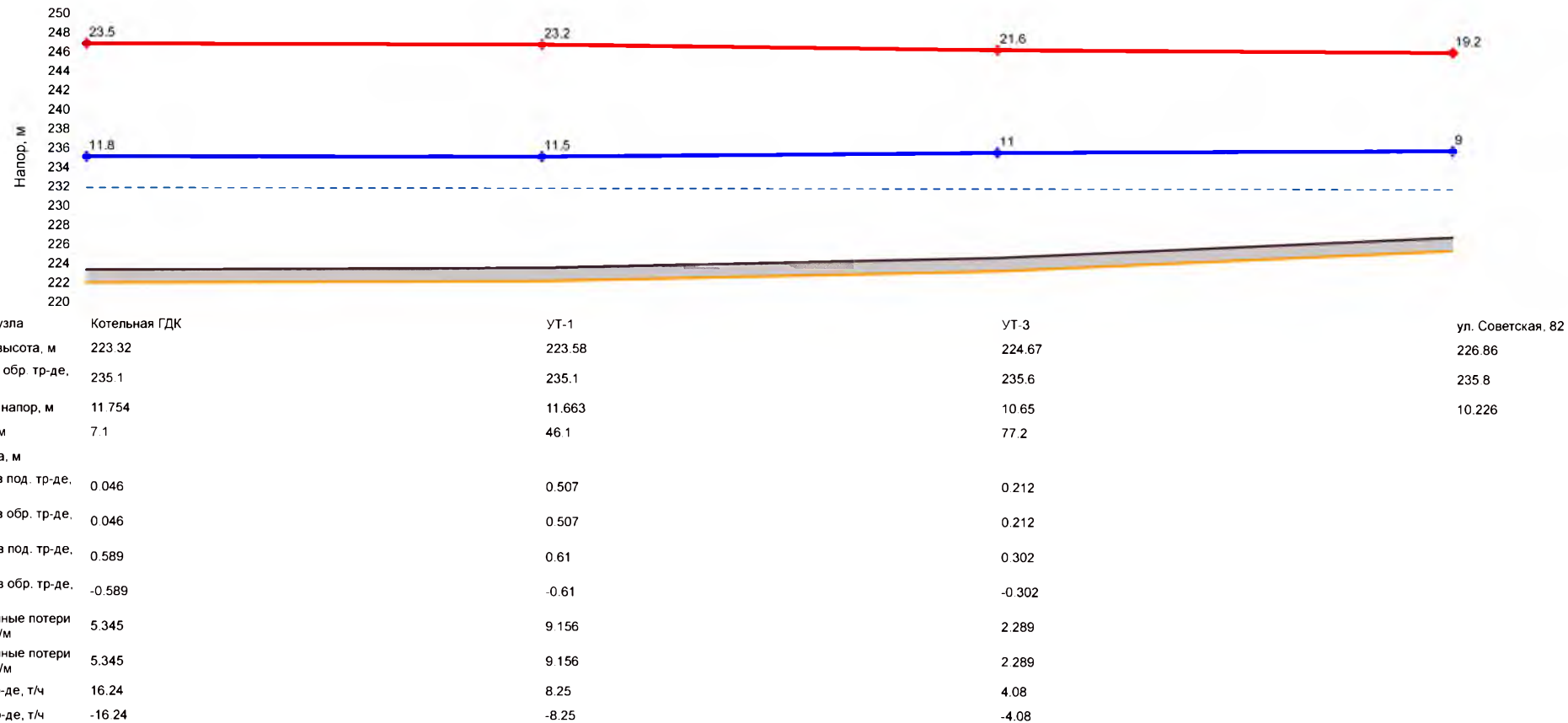
Рис. 20 – Пьезометрический график Котельной ГДК
