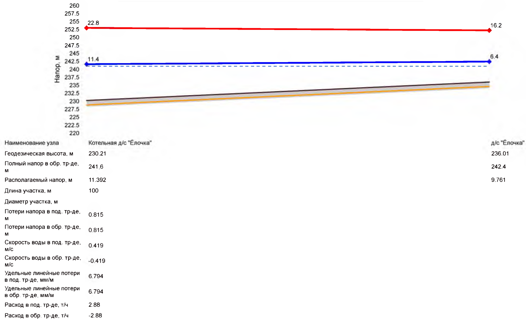
Рис. 13 – Пьезометрический график Котельной д/с «Ёлочка»
