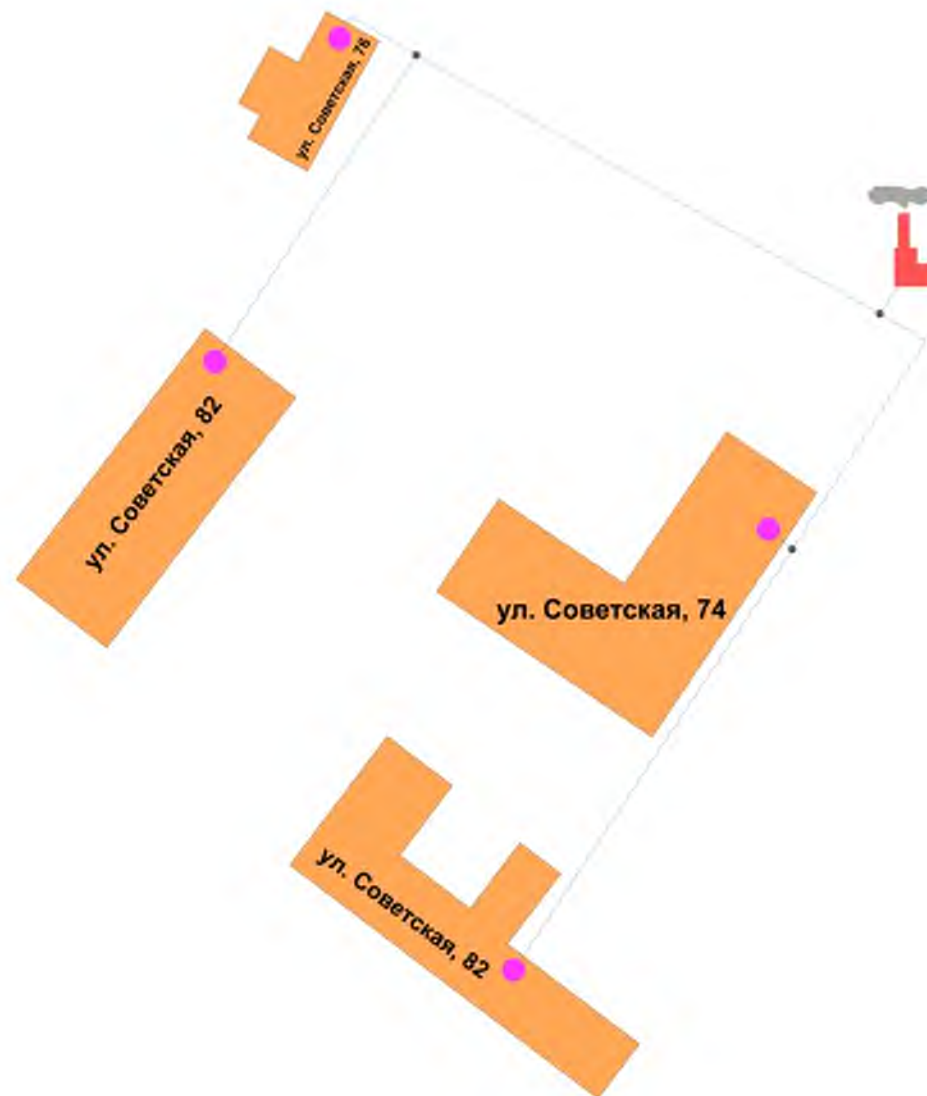
Рис.1 – Карта тепловых сетей котельной ГДК
