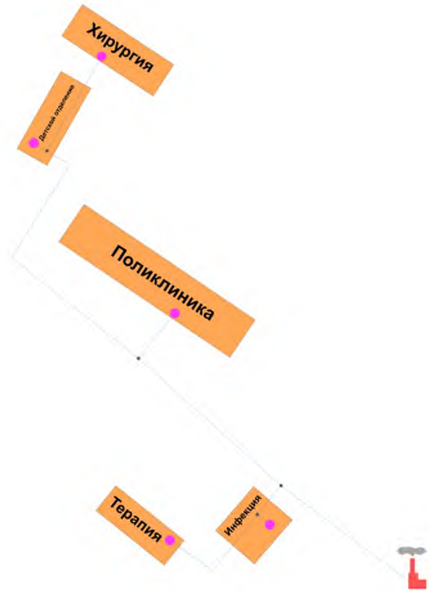
Рис. 10 - Карта тепловых сетей котельной ЦРБ
