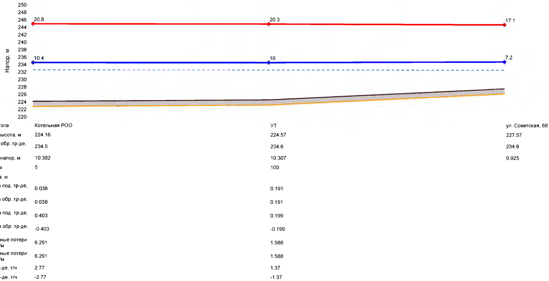
Рис. 18 – Пьезометрический график Котельной РОО
